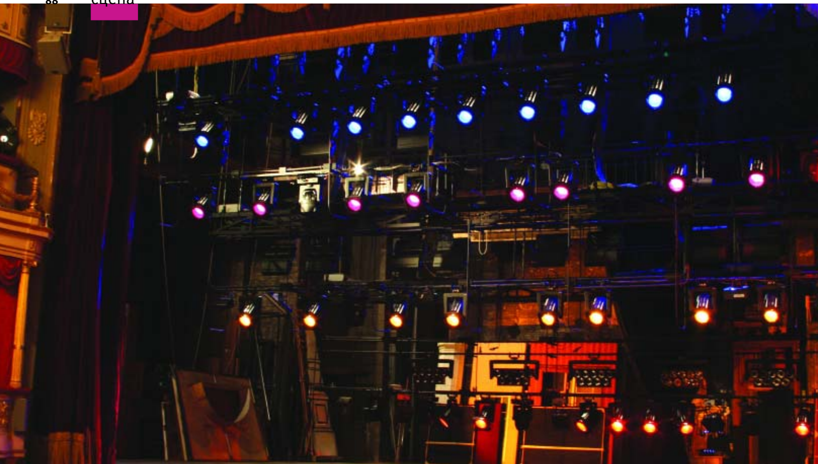
В ХОДЕ ПЕРВОГО ЭТАПА РЕКОНСТРУКЦИИ В 2006 ГОДУ, УСТАНОВЛЕНЫ: 48 ДИСТАНЦИОННО УПРАВЛЯЕМЫХ ПРОЖЕКТОРОВ НА БАЗЕ ЛИРЫ COMANDOR-E, СВЕТИЛЬНИКА ARENA 2500 PC ФИРМЫ SELECON СО СКРОЛЛЕРАМИ SPECTRUM-E 10
