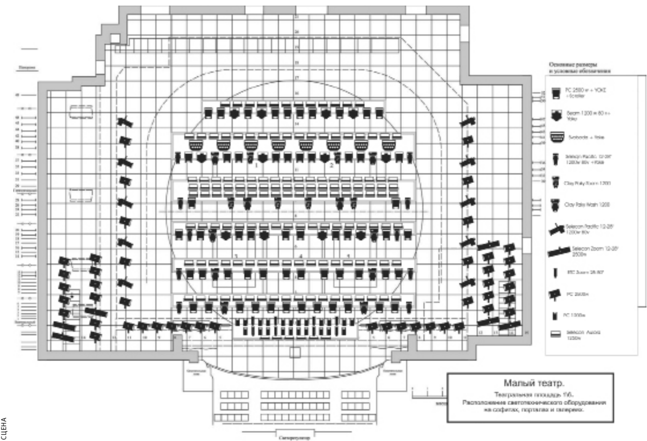
Схемы развеса светового оборудования
